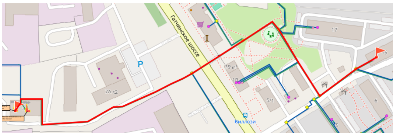
Рисунок 1.3.1. Трассировка выборочного участка теплосети для построения пьезометрического графика от котельной гп. Виллози до жилого дома № 15
